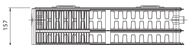
Тип 33 PLAN
